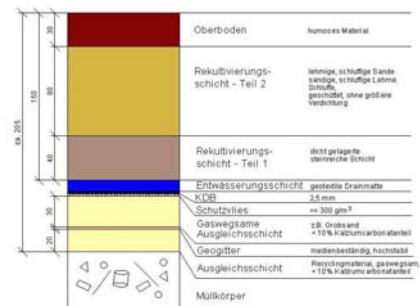
Regelschnitt 'Oberflächenabdeckung'
